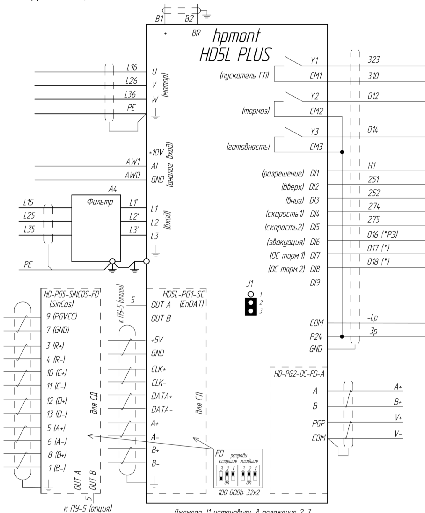
Рисунок 5.3 – Схема подключения к устройству управления УЛ
