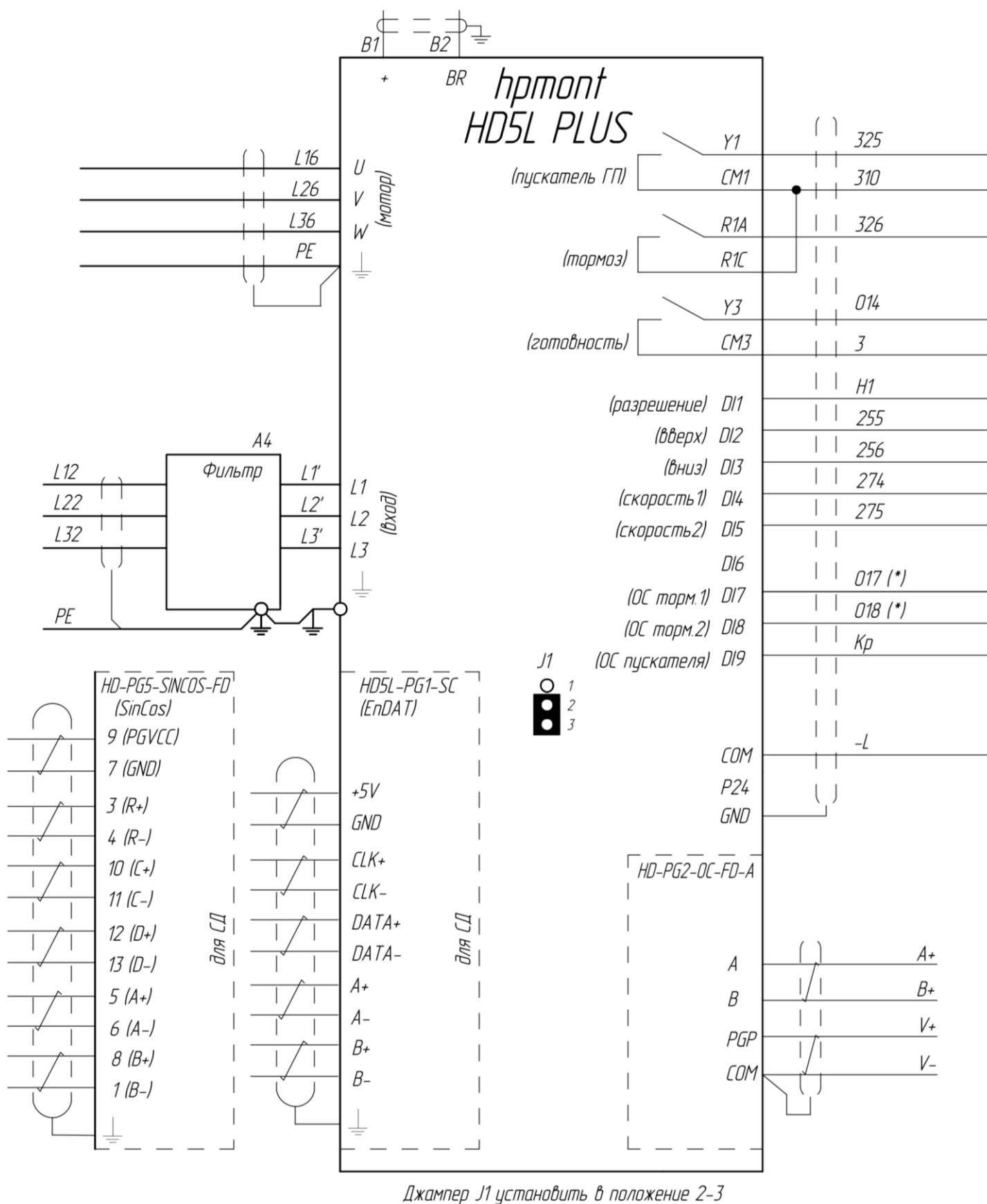
Рисунок 5.4 – Схема подключения к устройству управления УЛ для лифтов с ручными дверьми
