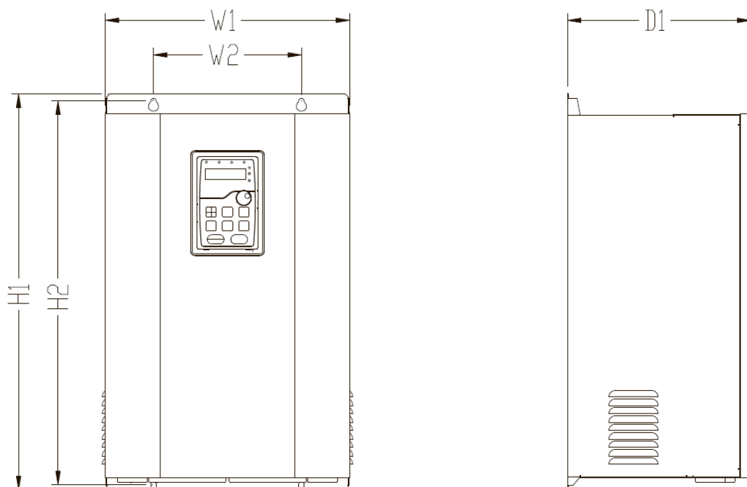
Рисунок 3.3 Конструкция 2
