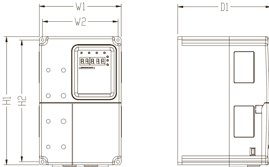
Рисунок 3.2 Конструкция 1
