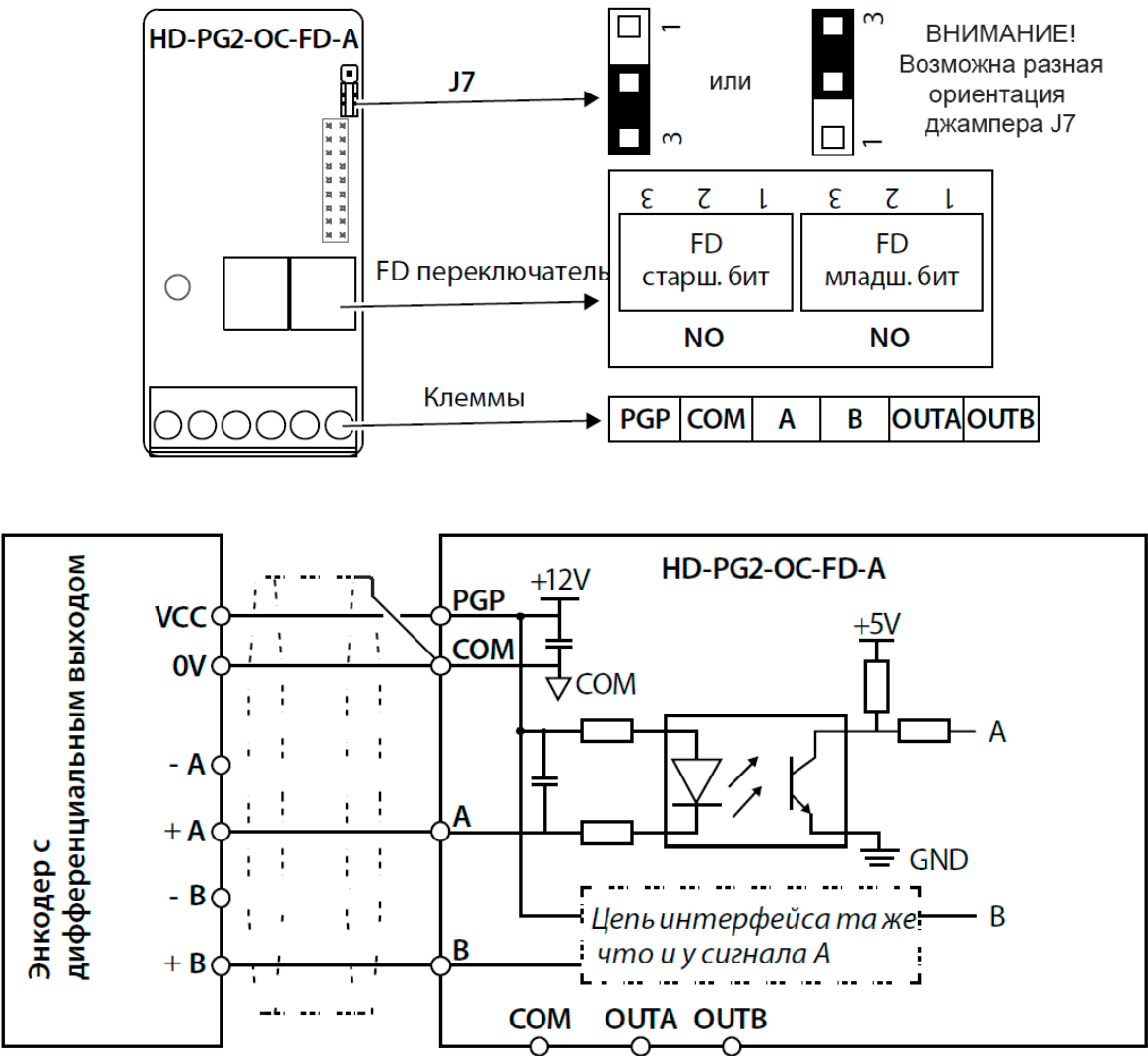
Рисунок 5.6 – Плата подключения энкодера HD-PG2-OC-FD-A
