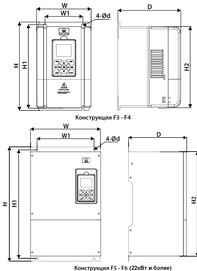
Рисунок 3.2 Габаритные размеры
