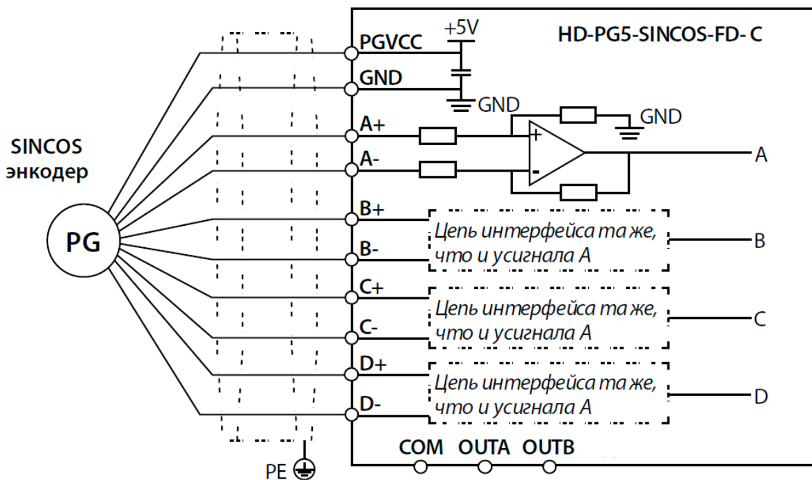
Рисунок 5.7 – Плата подключения энкодера HD-PG5-SINCOS-FD-C
