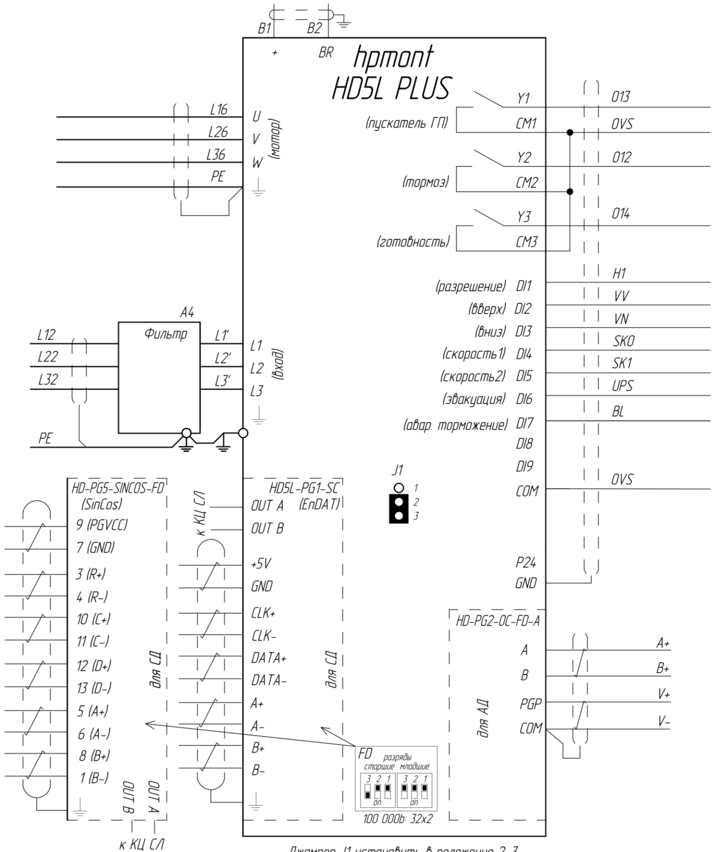
Джампер J1 установить в положение 2-3 Переключатели FD (делитель импульсов) на плате энкодера установить в соответствии с изображением FD
