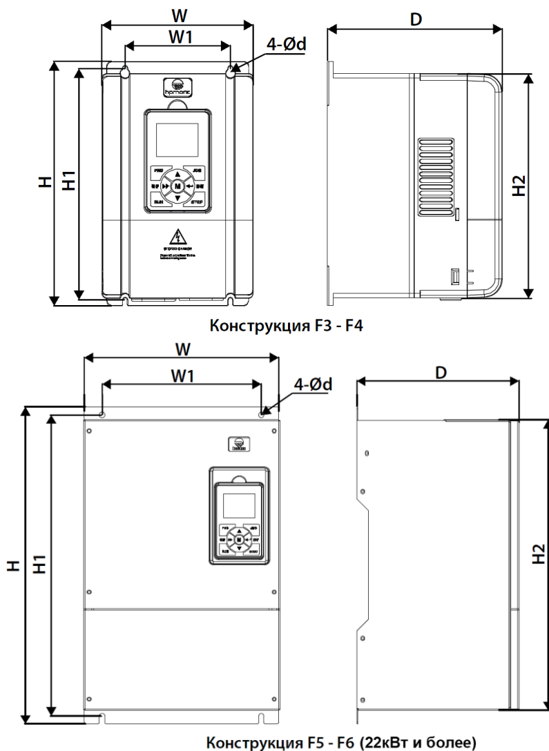
Рисунок 3.2 Габаритные размеры
