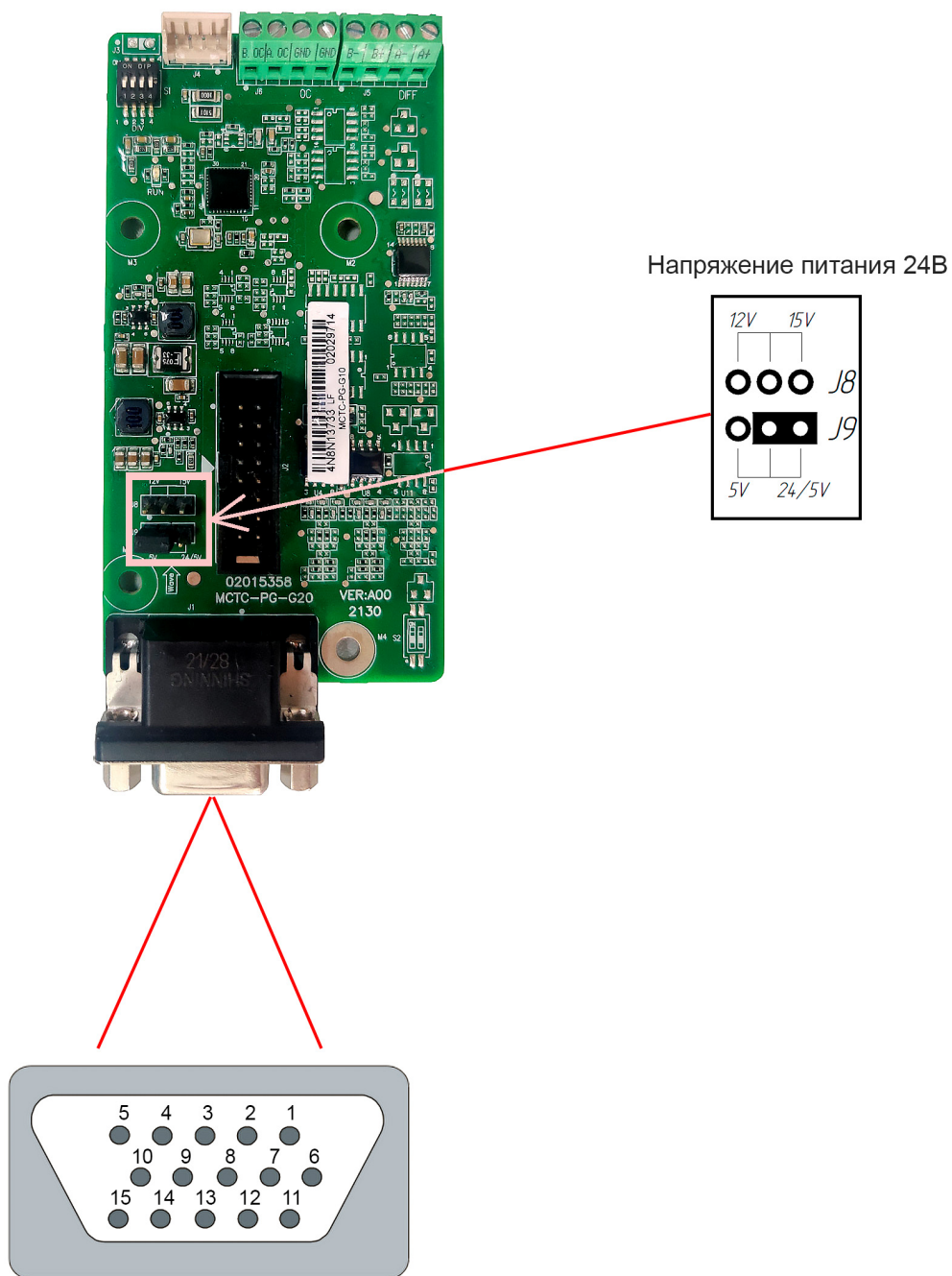
Рисунок 5.4 – Плата подключения энкодера МСТС-PG-G10
