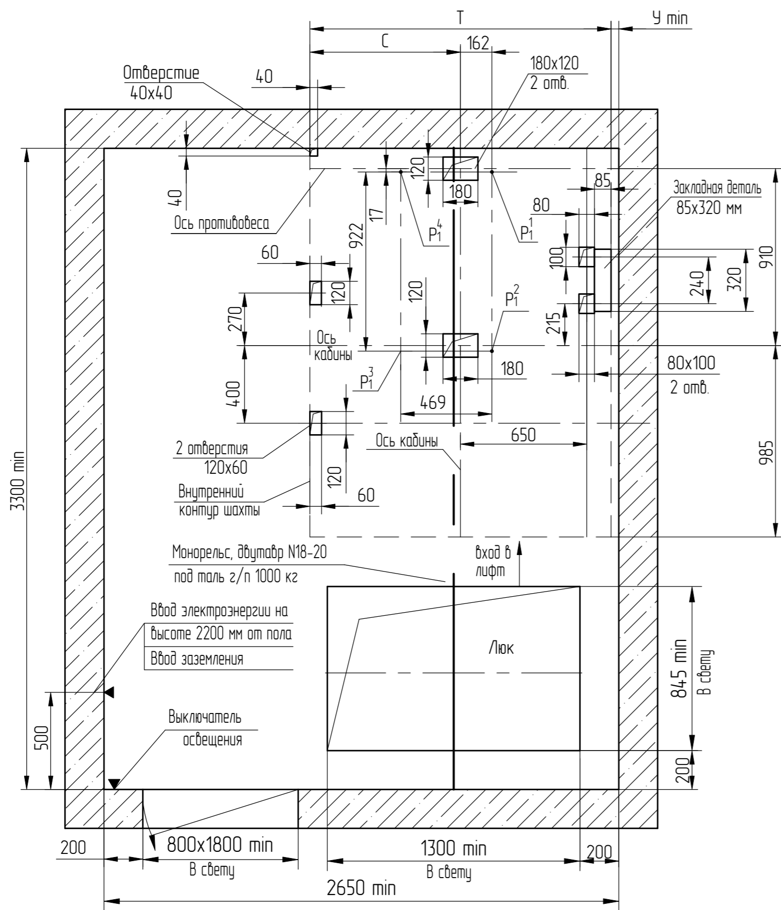
В-В (1:20) (1) Вариант I
