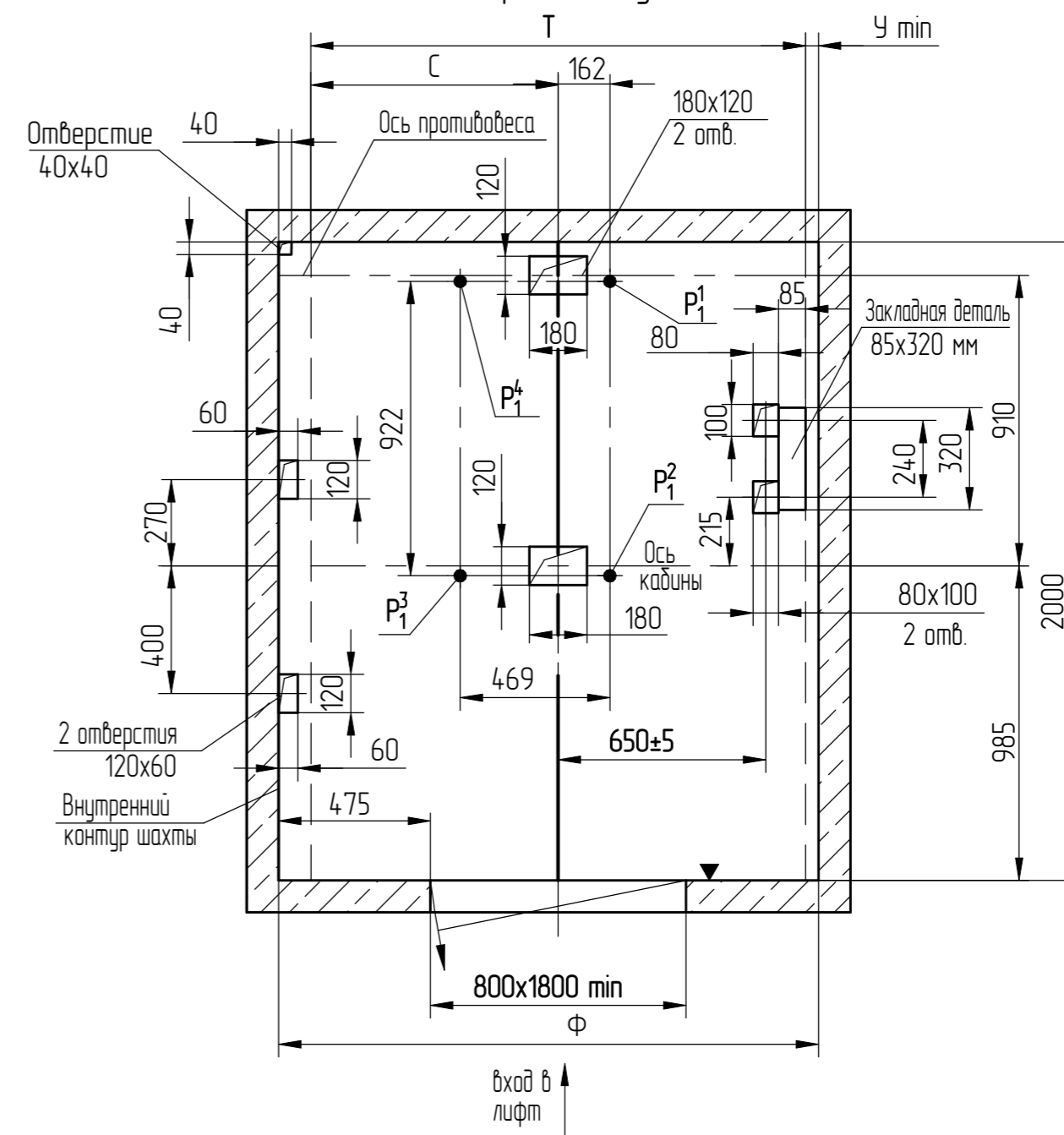
В-В (1:20) (1) Вариант II Малое машинное помещение (не рекомендуется)
