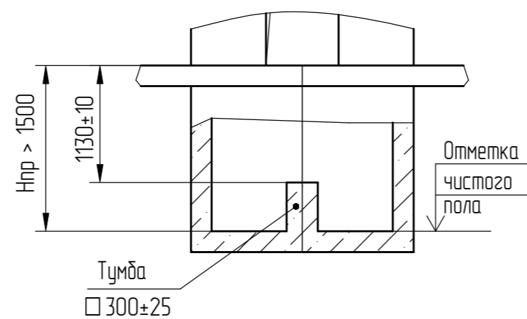
И (1) При глубине приямка H_{пр} > 1500 мм (не рекомендуется)
