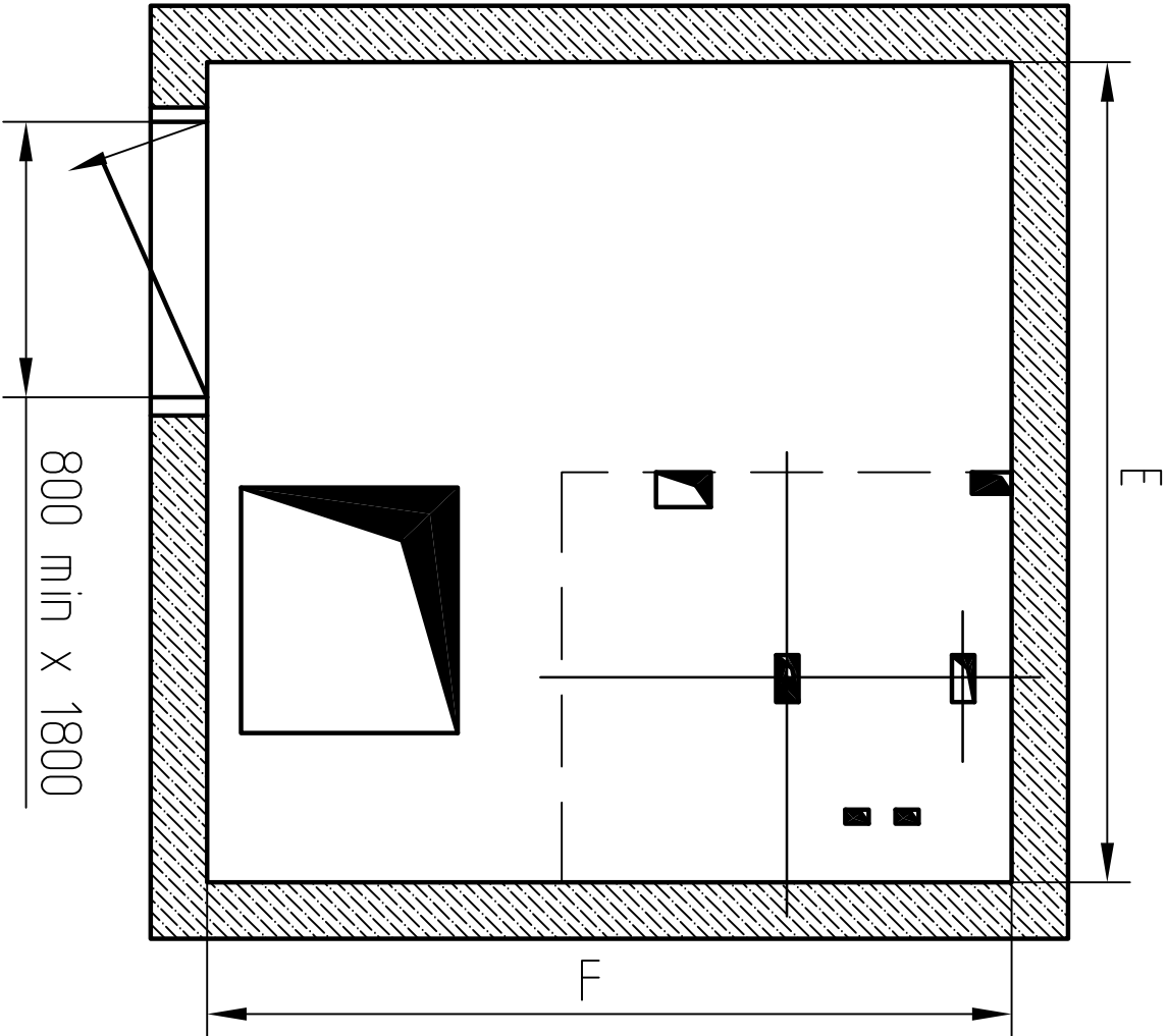
План шахты - вариант 1 План машинного помещения
