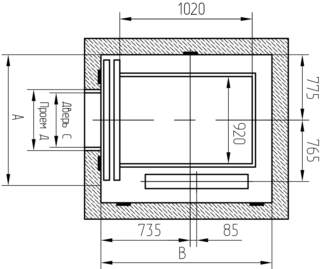
План шахты - вариант 1 План машинного помещения
