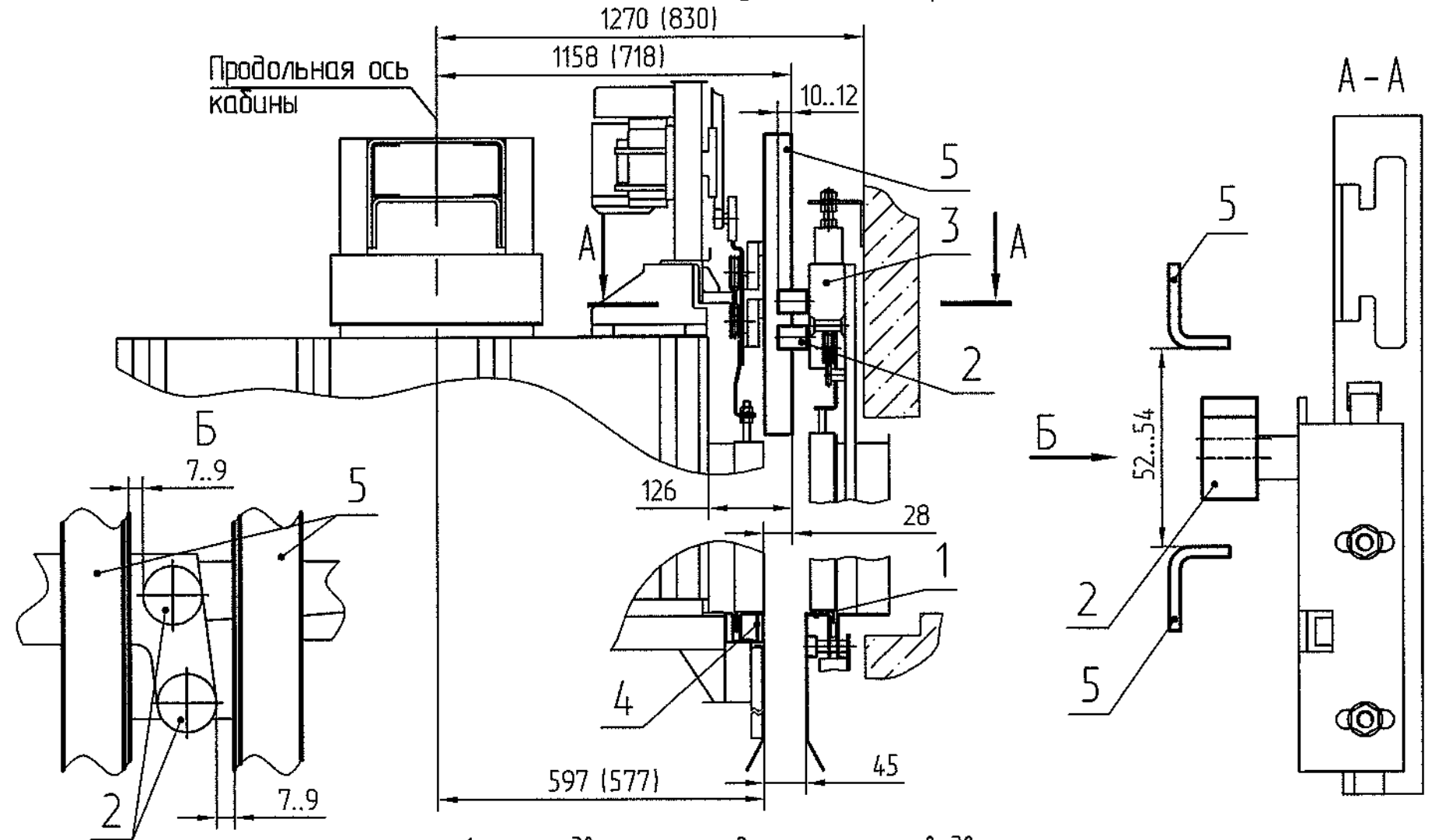
1- порог двери шахты; 2- ролики замков двери шахты; 3- балка дверей шахты; 4- порог двери кабины; 5- отводка привода дверей кабины Рисунок Е.15
