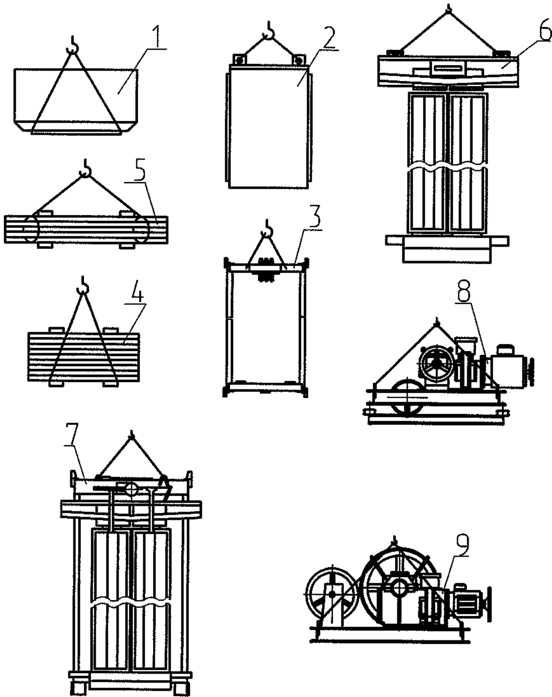
1- Ящика; 2- шкафа; 3- каркаса противовеса; 4- грузоб противовеса; 5- пакета направляющих; 6- дверей шахты; 7- кабины; 8, 9- лебедок.
