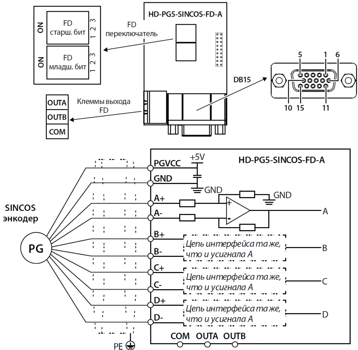
Рисунок 5.7 – Плата подключения энкодера HD-PG5-SINCOS-FD-A
